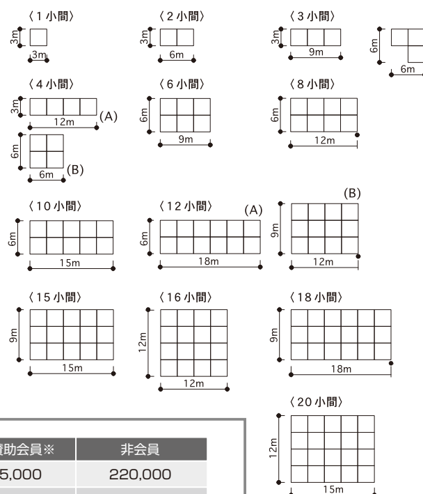
一般小間の形態図
